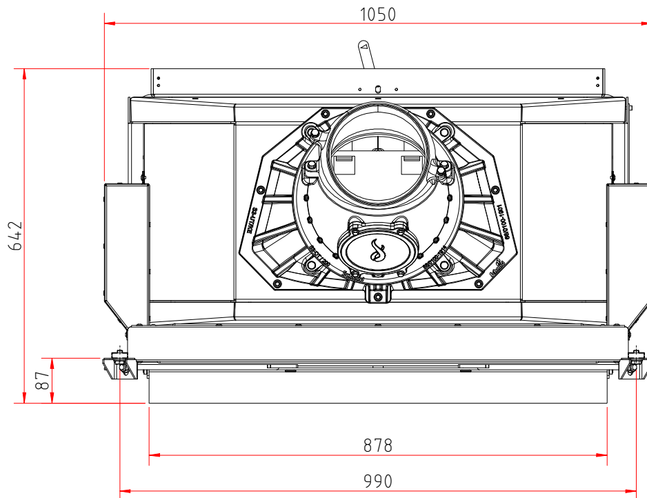
Draufsicht M 1:10
