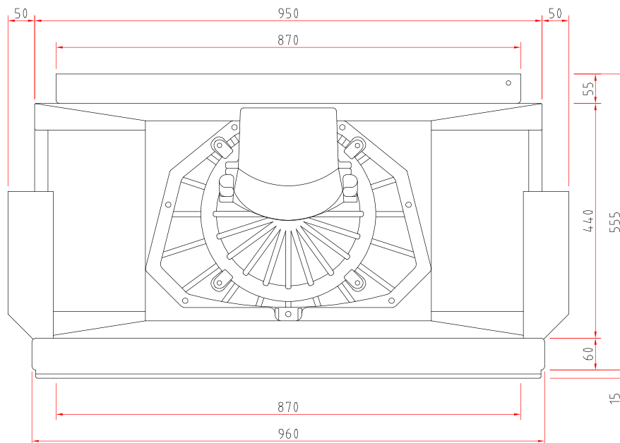
Draufsicht M 1:10
