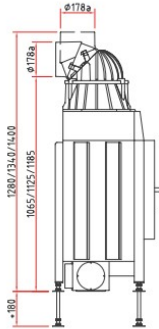
Seitenansicht M 1:20
